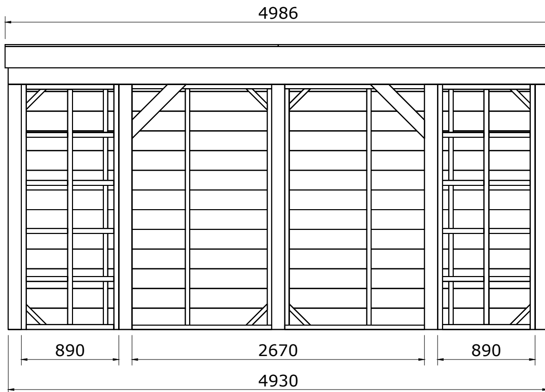
Voor aanzicht
