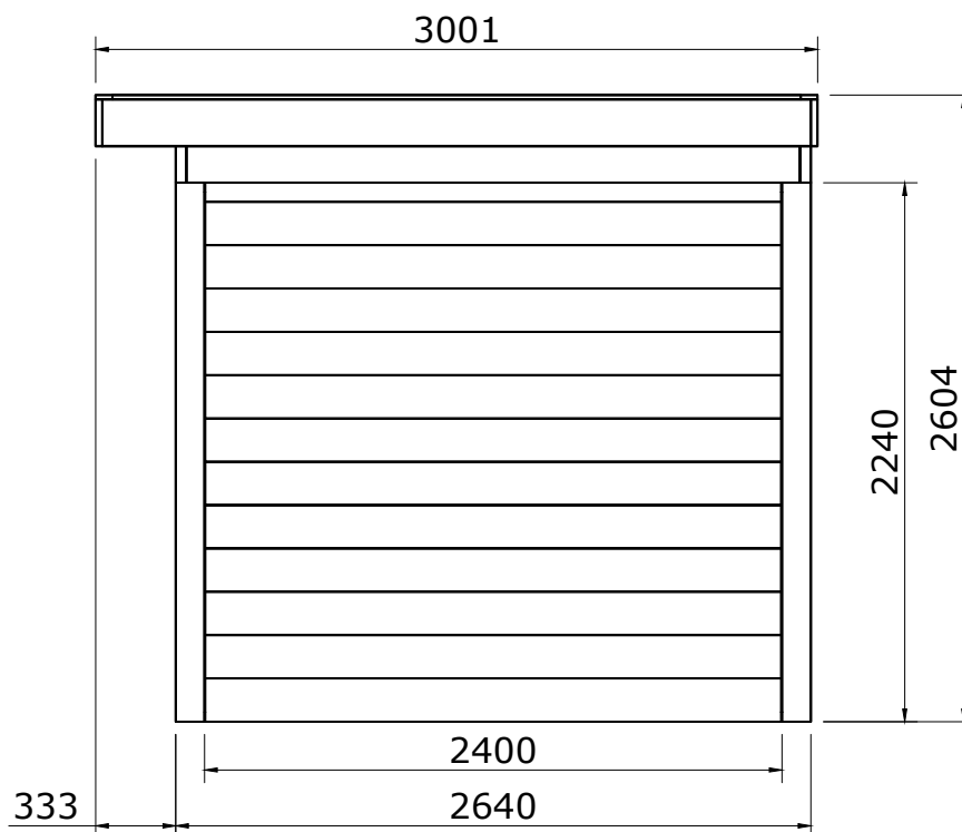
Rechter zijaanzicht
