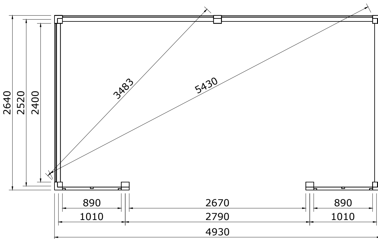
Palenplan
